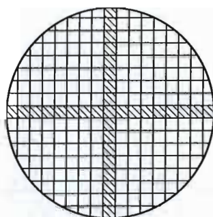
网孔以不规则间隔分布在所有的直径上,测量纬向和经向尺寸,每个网孔只测一个方向
